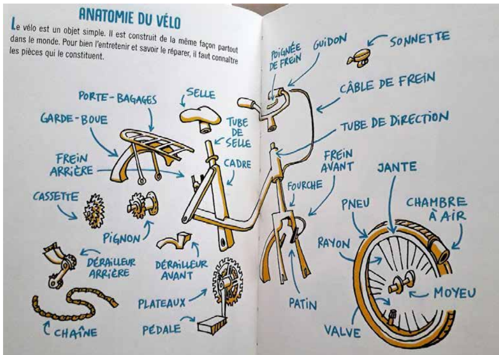
Mission vélo anatomie du vélo ffl © Velo101
